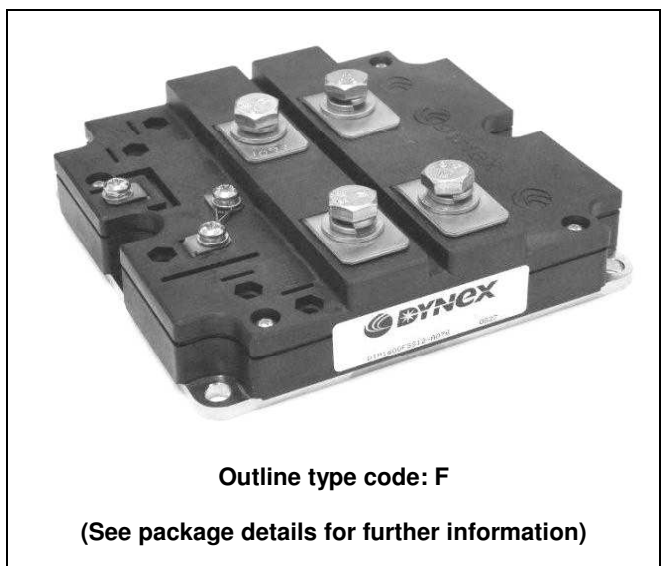
Fig. 2 Module Package
