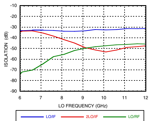
Isolation LO/IF, LO/RF, 2LO/IF
