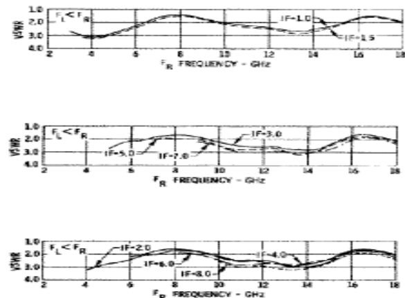
R-Port VSWR LO @ +13 dBm
