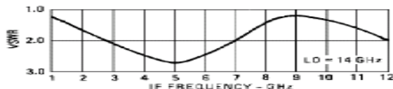
I-Port VSWR
