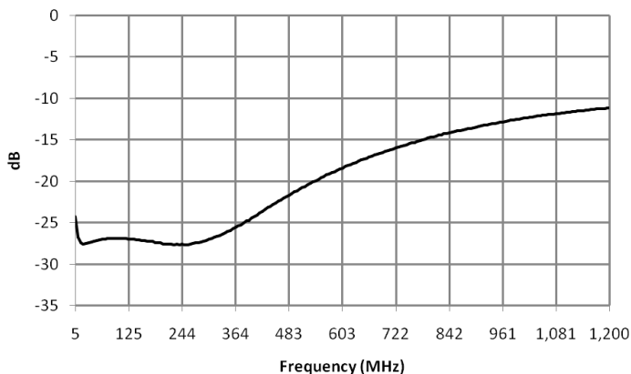
MABA-011029 input_return_loss_p1
