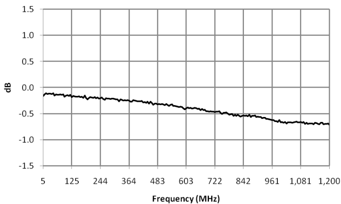
MABA-011029 amplitude_balance
