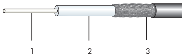
Fig. 2: SUCOFORM_141_CU_LSFH-01
