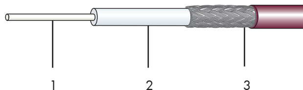
Fig. 2: SUCOFORM_141_CU_PE
