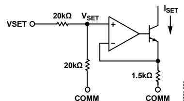
Figure 25. VSET Interface
