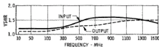
VSWR
