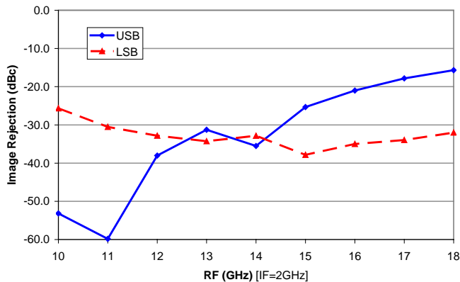
XU1005-QD, Image Rejection (dBc)
