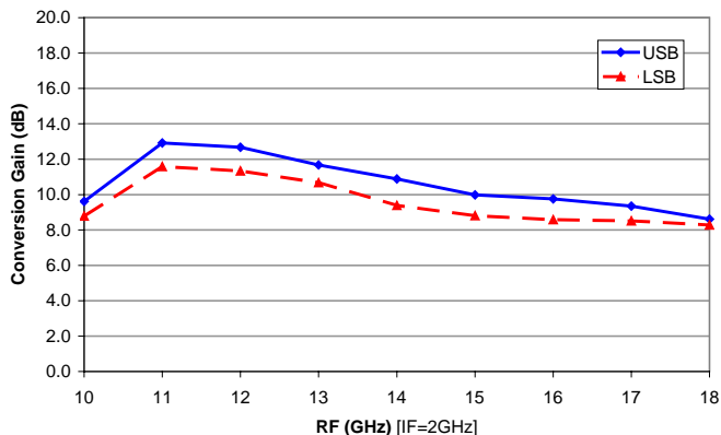
XU1005-QD, Conversion Gain (dB)
