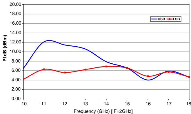
XU1005-QD P1dB Compression
